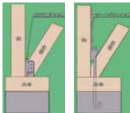
筋交金物 ホールダウン金物
