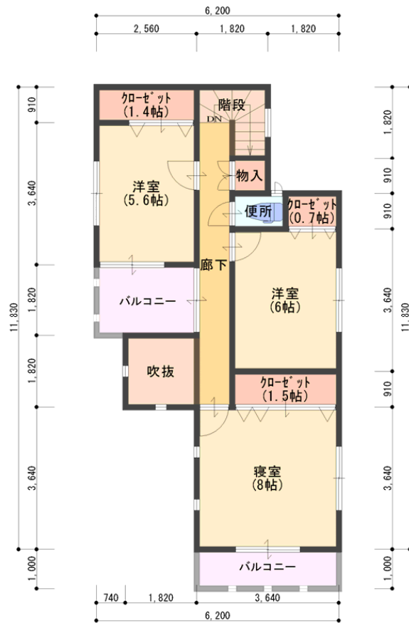
2階平面図
